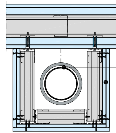
RAUPIANO PLUS 2x 12,5 mm Diamant
